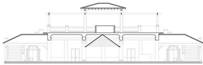
SECCION LONGITUDINAL
