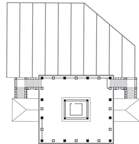
PLANTA MIRADOR
